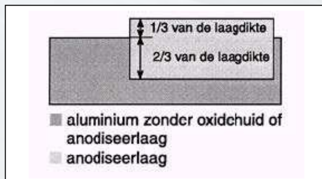
Figuur 2 Schematische voorstelling anodiseer-laag
