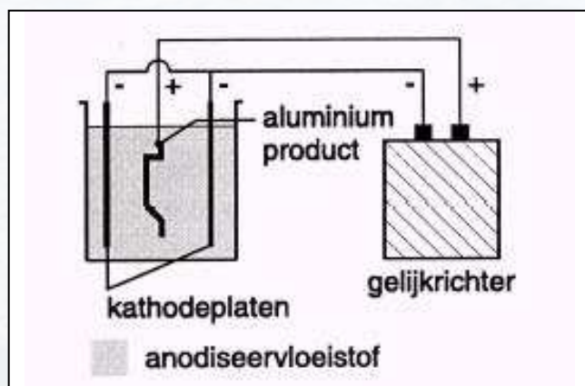
Figuur 1 Principe van anodiseren
